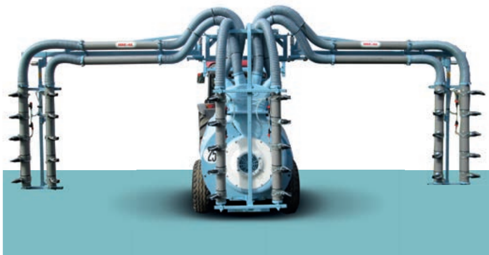
● Hidraulikus karok 3 teljes sorra - 6 diffúzor 5 fuvókával
